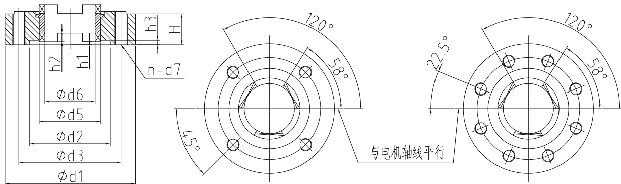
XZA系列连接尺寸（JB2920标准）
